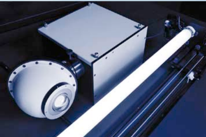
Qualitätsmanagement: Spektralmessung einer Einzellampe
